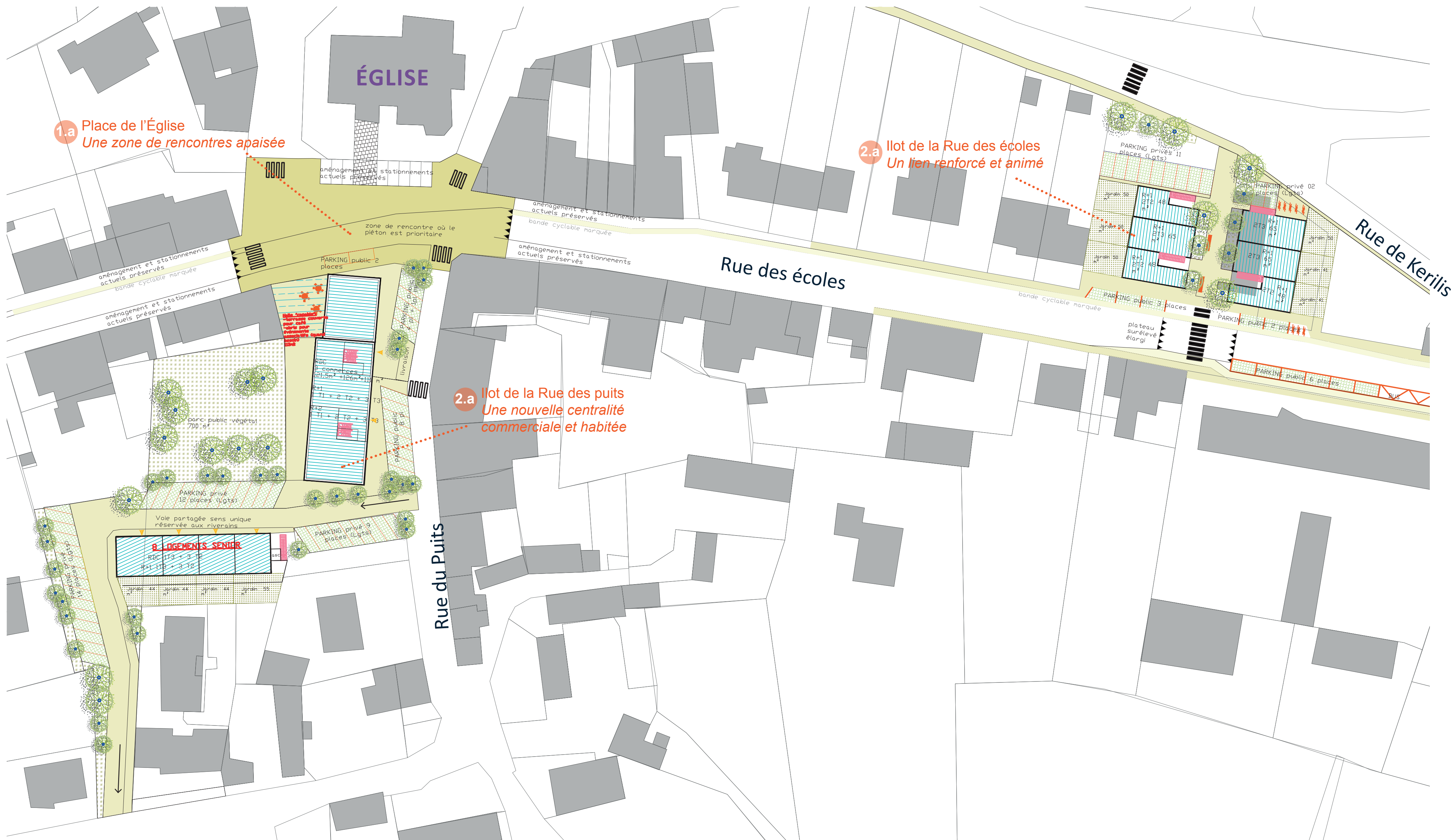
Plan masse - échelle 1 : 500
